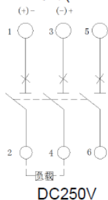
接线图(NDM3ZB-125)
