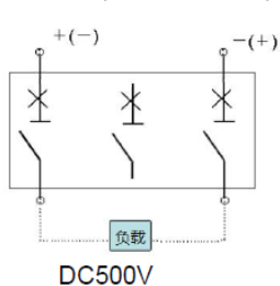
接线图: (NDM3Z-125)
